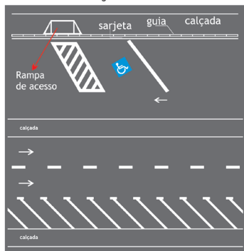
Estacionamento em ângulo
