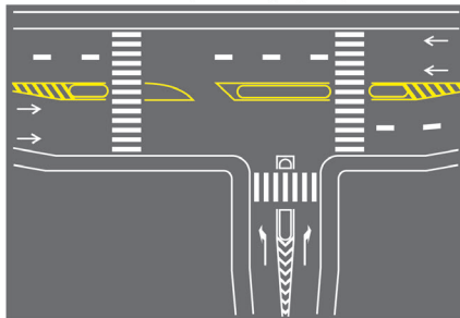
Ilhas de canalização e refúgio para pedestres
